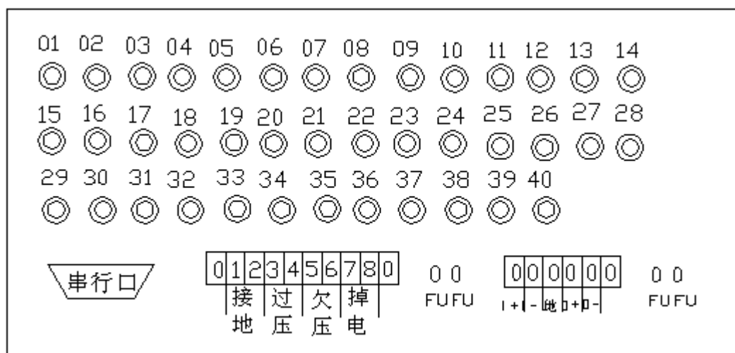
图 5B 监测路数小于等于 40 路的装置后面板图
