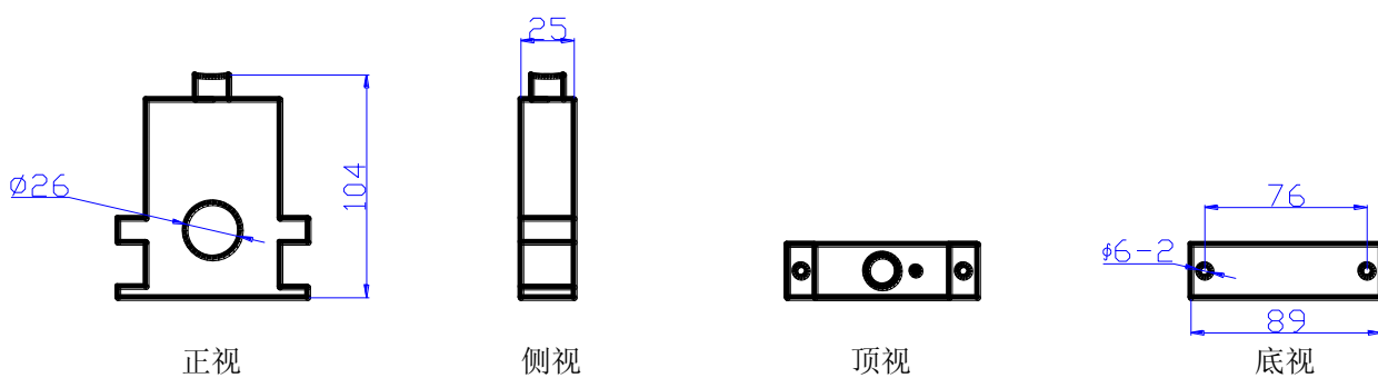
附图 2：传感器尺寸(单位：mm)
