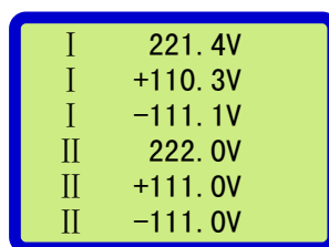
两段母线画面
