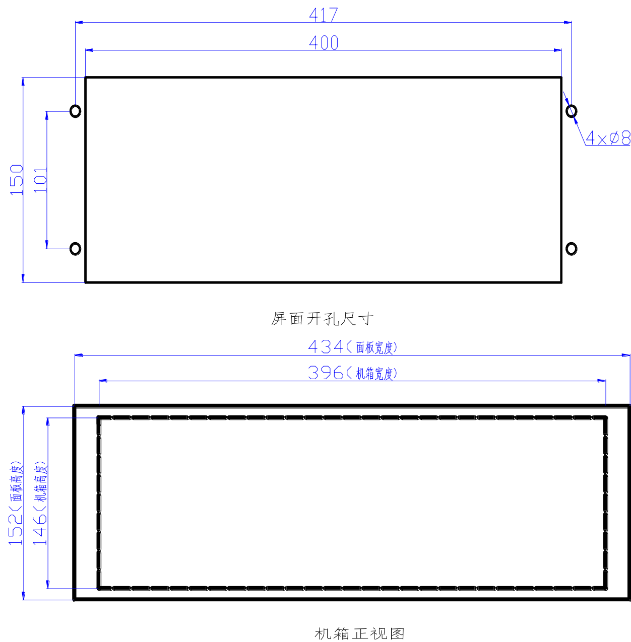
附图 1：装置机箱尺寸及屏面开孔尺寸(单位：mm)
