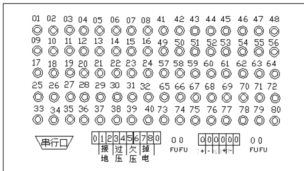
图 5A 监测路数为 80 路的装置后面板图
