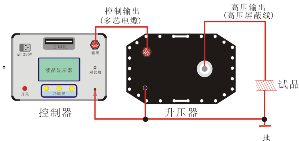
图 4 (连线图)
