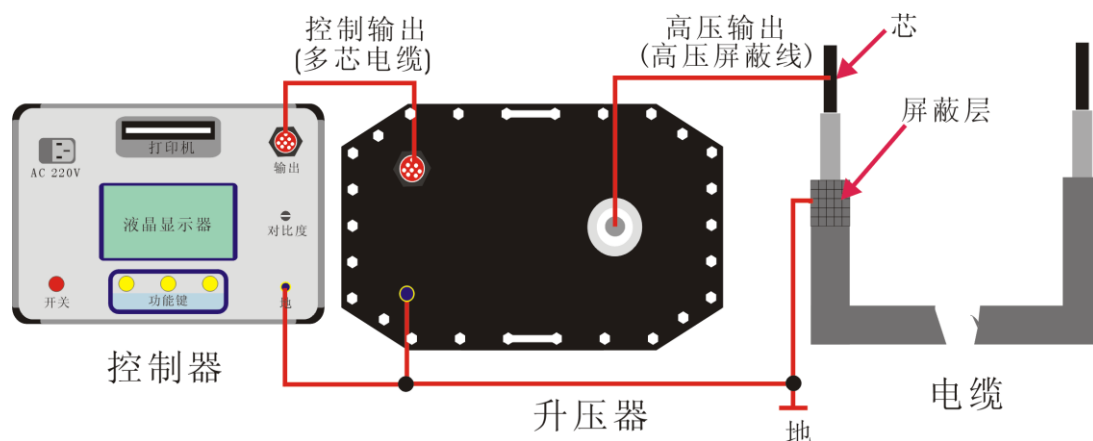
图 13 单相测量连线图
